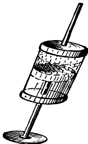
Рис. 2. Шприц Жане для визначення концентрації \text{CO}_2 за Д.В. Прохоровим.
