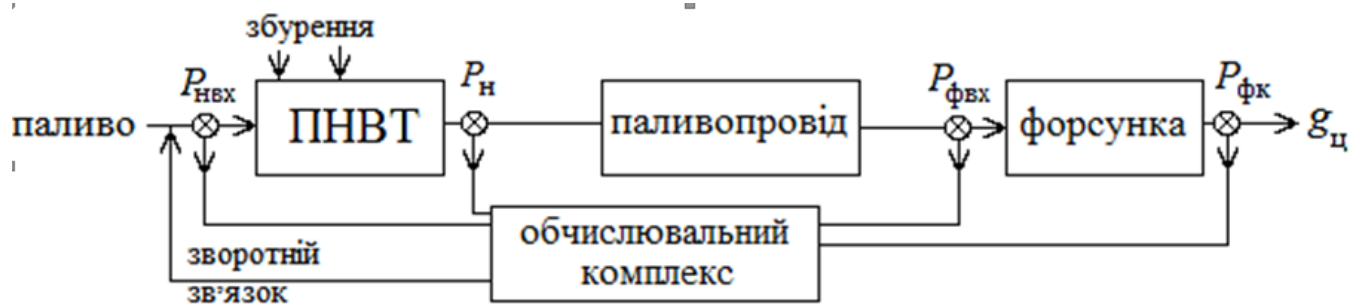
Рис. 1. Система контролю за впорскуванням палива у судновому дизельному двигуні:
