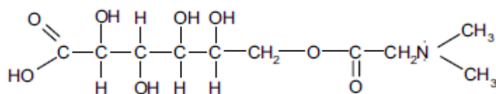
Пангамова кислота
