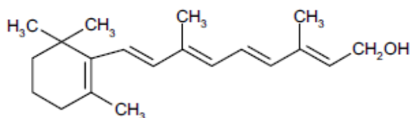
Вітамін А
