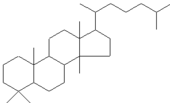
Ланостан
