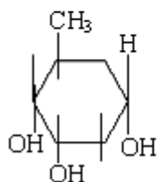
Д-дигітоксоза
