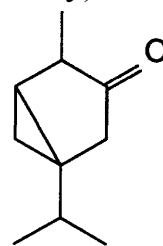
туйон
