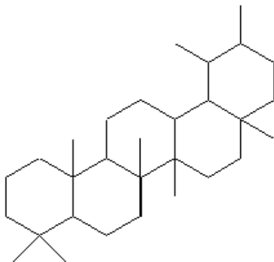
Урсан
