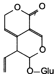
генціопікросид (генціопікрин)
