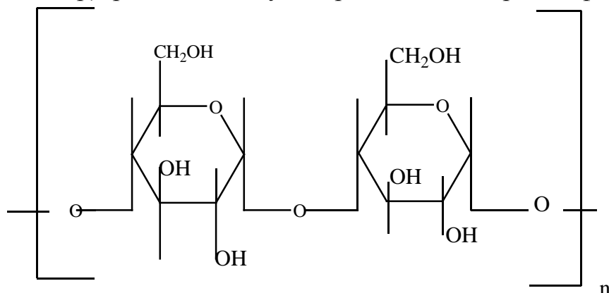
Амілоза (фрагмент)
