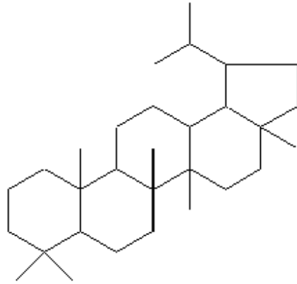
Лупан
