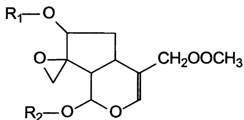
дигідровалтрат
