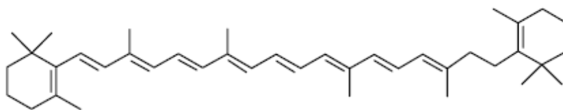
β-Каротин
