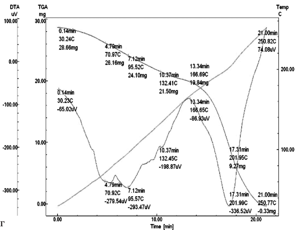
Рис. 1. Дериватограми адемолау (А), пластифікатора – гліцерину (Б), мукоадгезивного компоненту гідроксиетилцелюлози (В) та консерванта бензалконію хлориду (Г)
