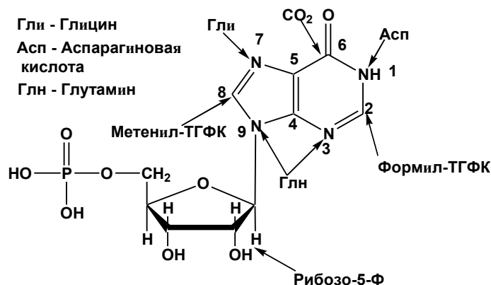
Рис. 5. Соединения, участвующие в синтезе ИМФ.
