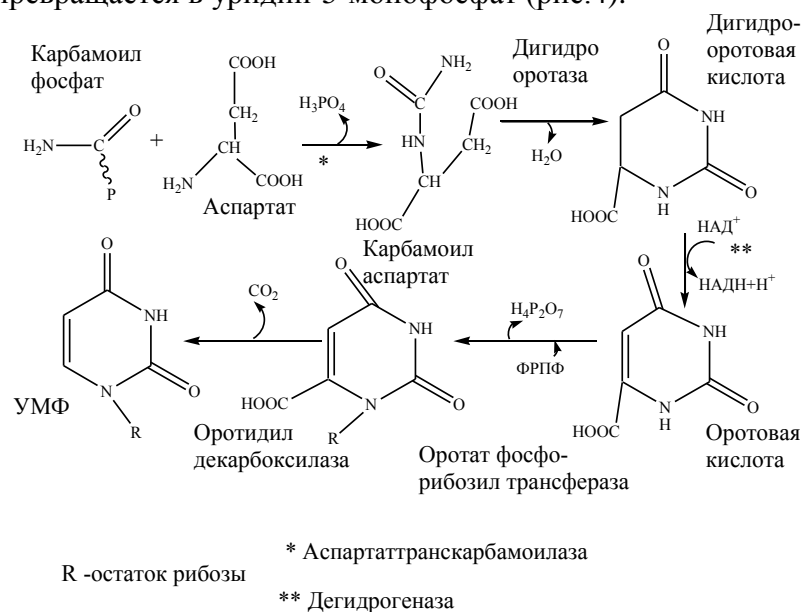
Рис. 4. Синтез уридин-5-монофосфата
