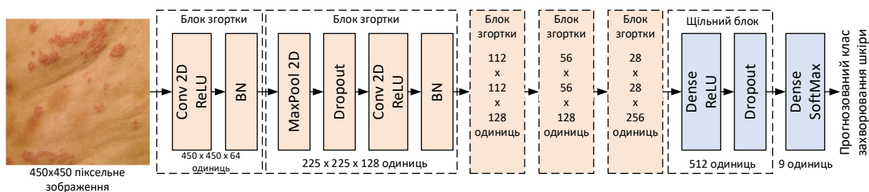
Рисунок 1 – Архітектура ЗНМ, що використовується для класифікації захворювань шкіри
