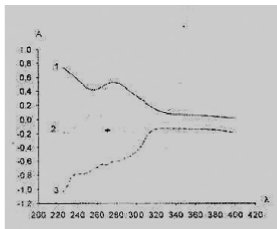
Рис. 2 . Спектри поглинання:
